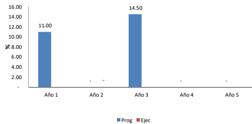
Aplicación de incrementos tarifarios agua potable
